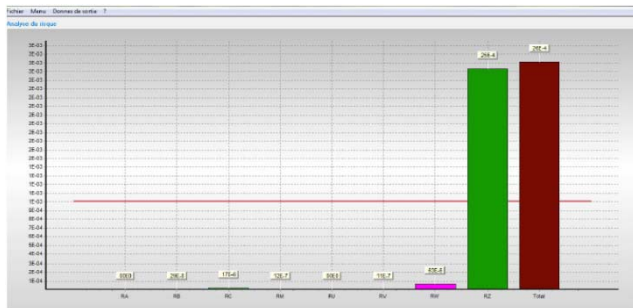
Risque de perte de production calculé avec le logiciel Jupiter
