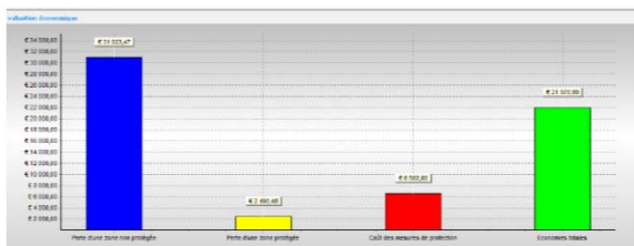
Intérêt économique de la protection par paratonnerre
